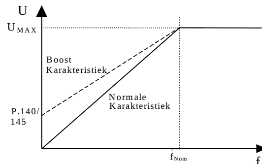
Afbeelding 2 Boostkarakteristiek
