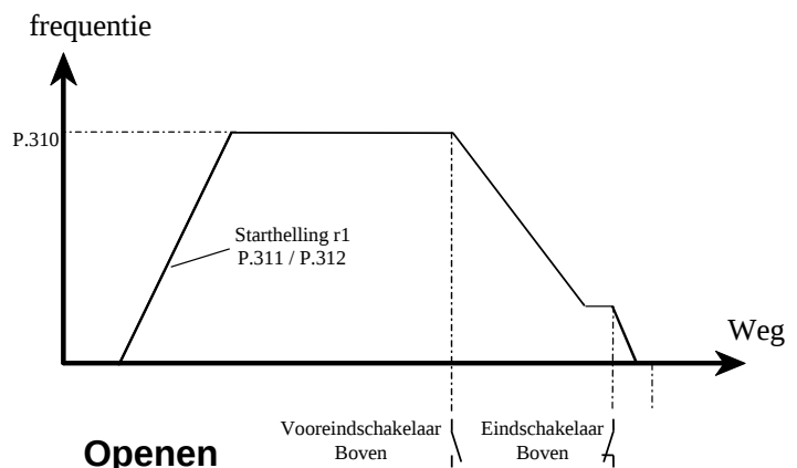
Afbeelding 8 Starthelling OPEN-beweging
