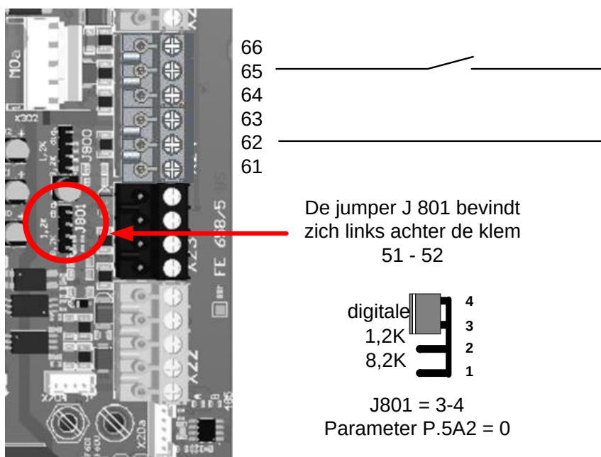
Afbeelding 15: Aansluiting van een weerstands- veiligheidsstrip
