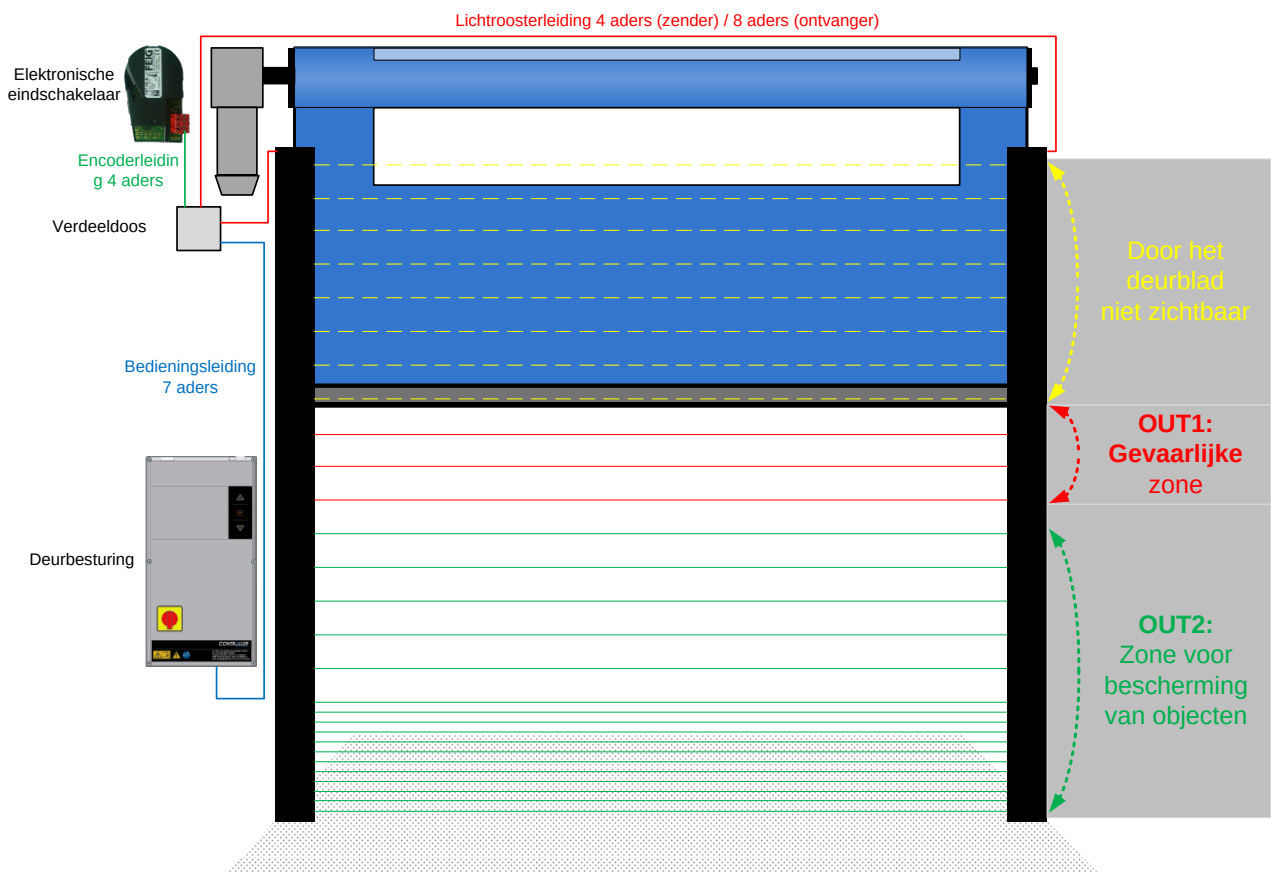
Afbeelding 16: Montage van de TST LGB
