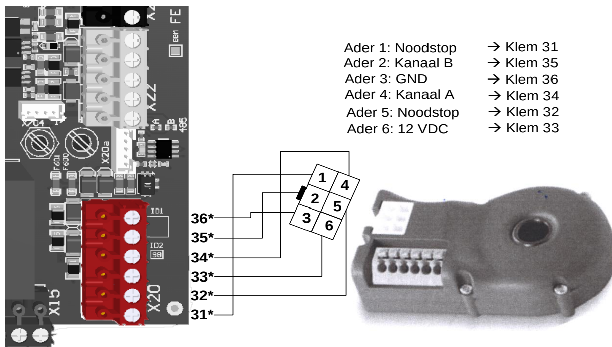
Afbeelding 20: Aansluiting absolute encoder DES
