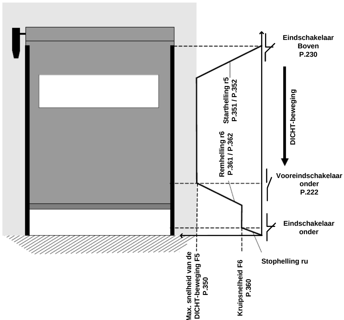
Afbeelding 40: DICHT-beweging met frequentie-omzetter
