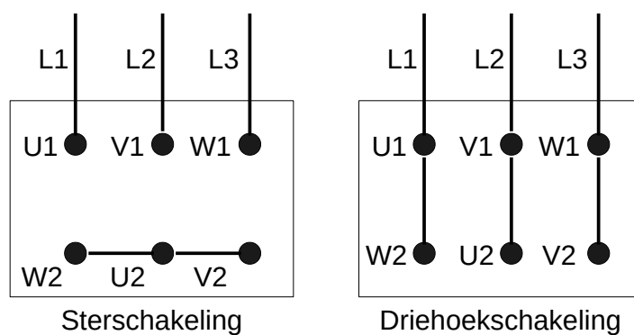
Afbeelding 38: Ster- / driehoekschakeling
