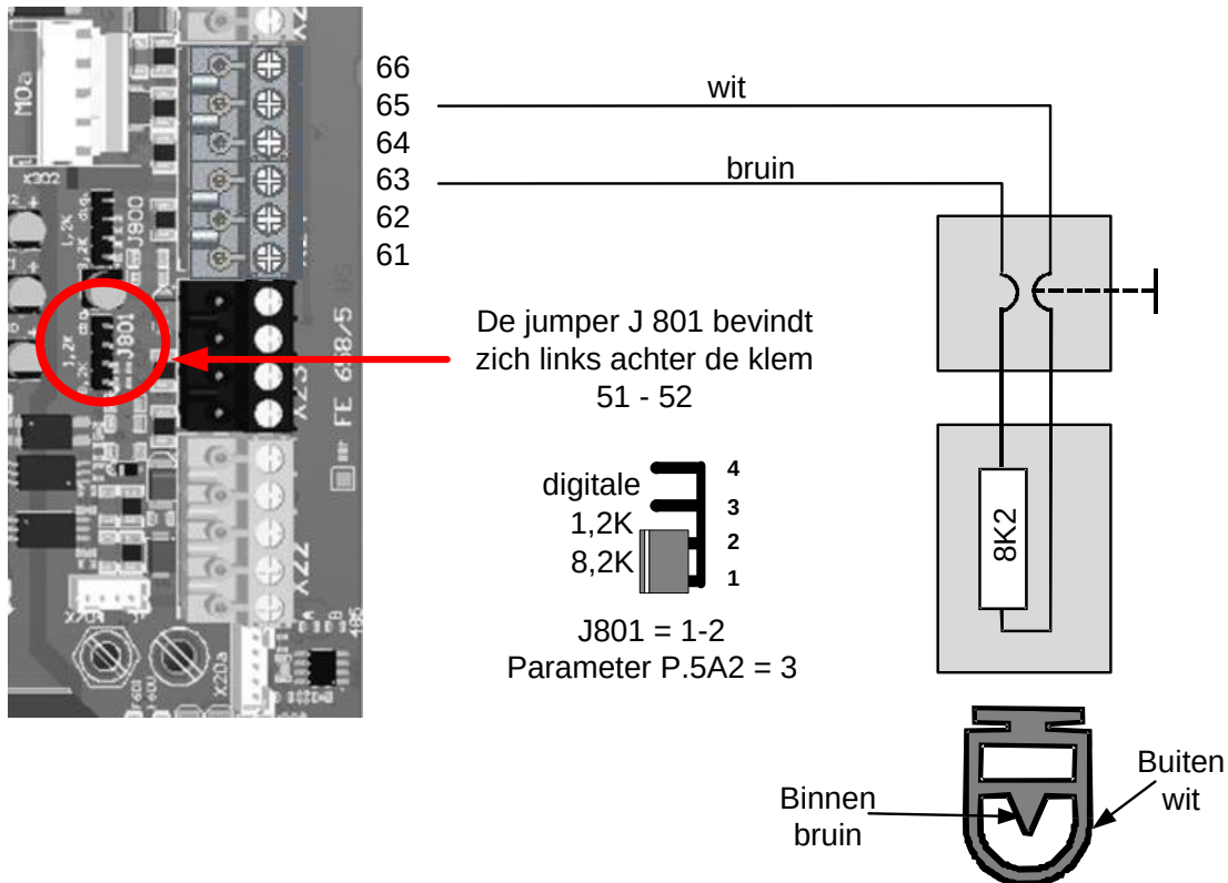
Afbeelding 14: Aansluiting van een weerstands- veiligheidsstrip
