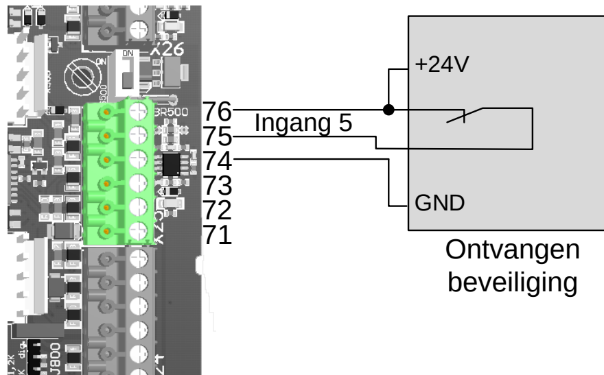
Afbeelding 22: Aansluiting foto-elektrische beveiliging
