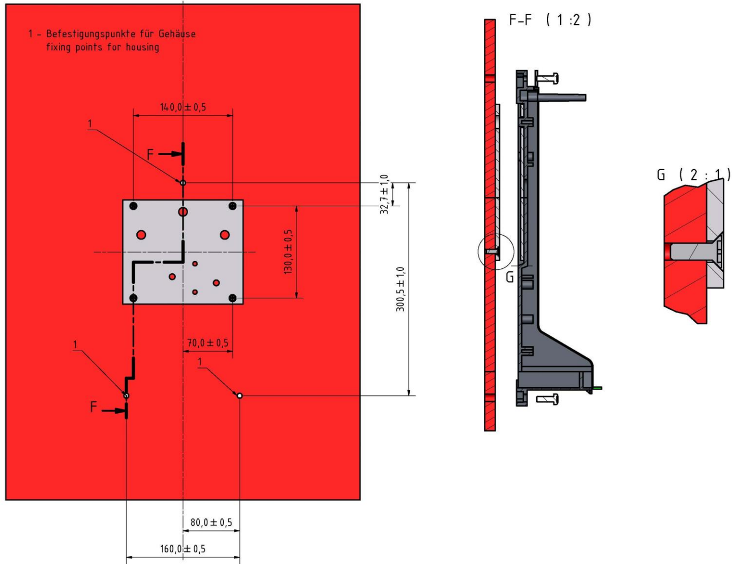
Afbeelding 5: Boorschema voor extra koellichaam en besturing
