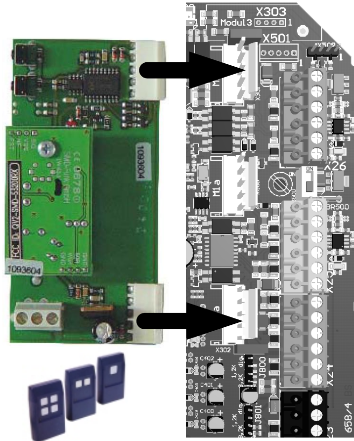
Afbeelding 27: Radio-steekontvanger
