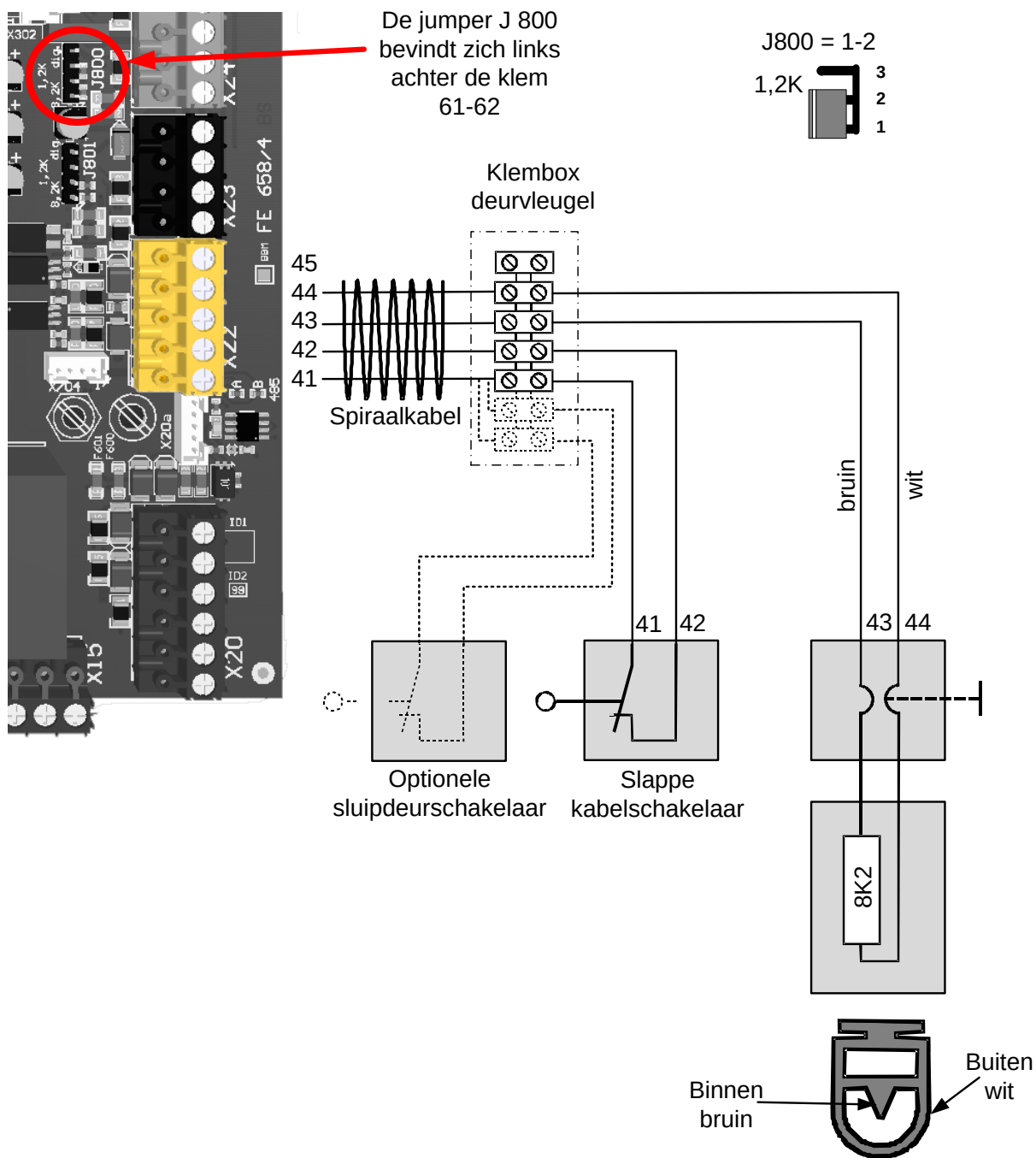
Afbeelding 12: Aansluiting van een weerstands- veiligheidsstrip
