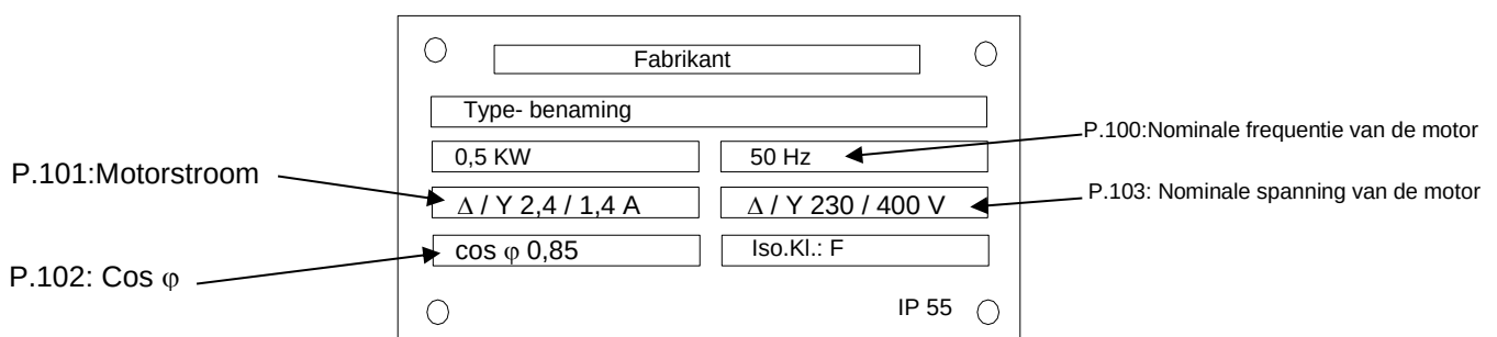
Afbeelding 37: Voorbeeld motortypeplaatje (afb. soortgelijk)
