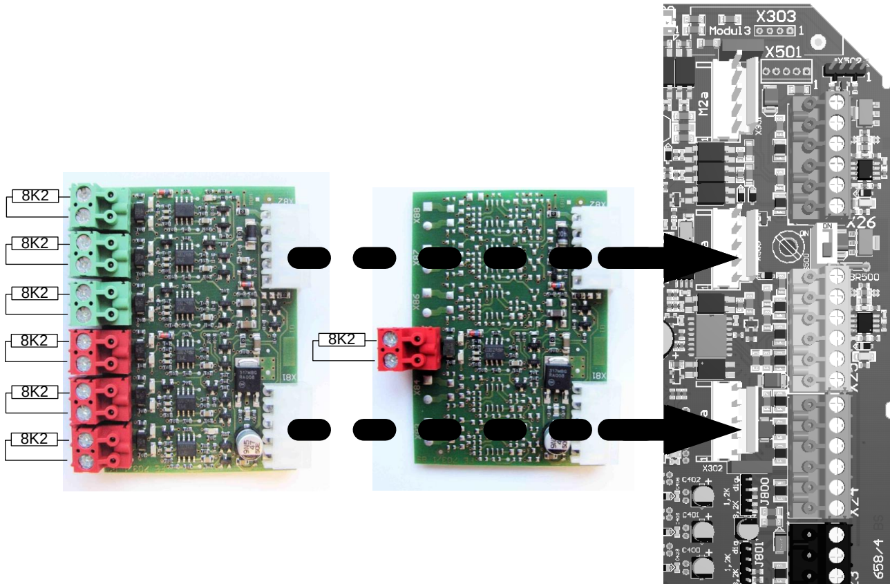
Afbeelding 30: Veiligheidsstripanalyse
