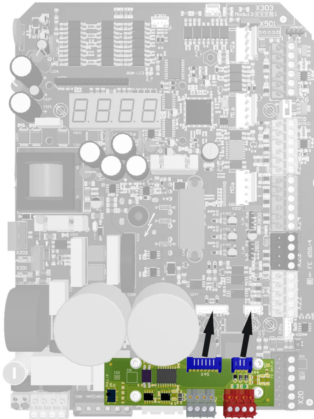
Afbeelding 32: Interfacekaart RFuXFCOM
