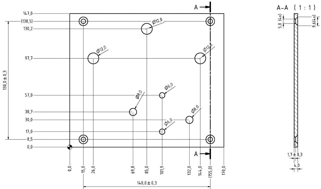
Afbeelding 4: Extra koellichaam
