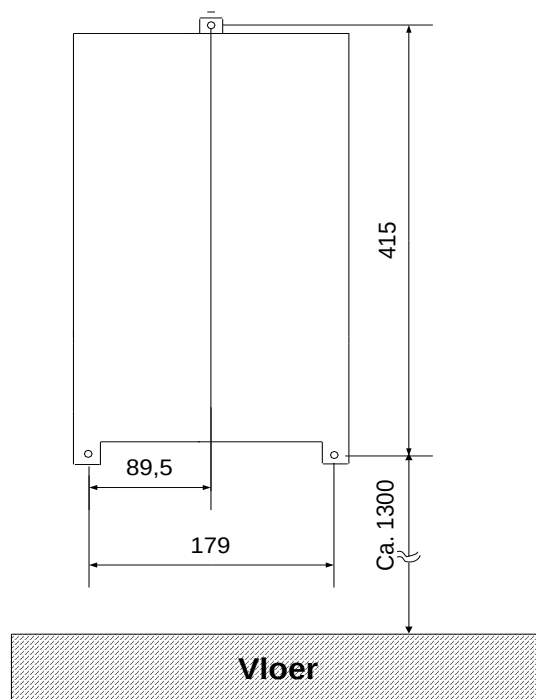
Afbeelding 7: Boorschema van grote behuizing
