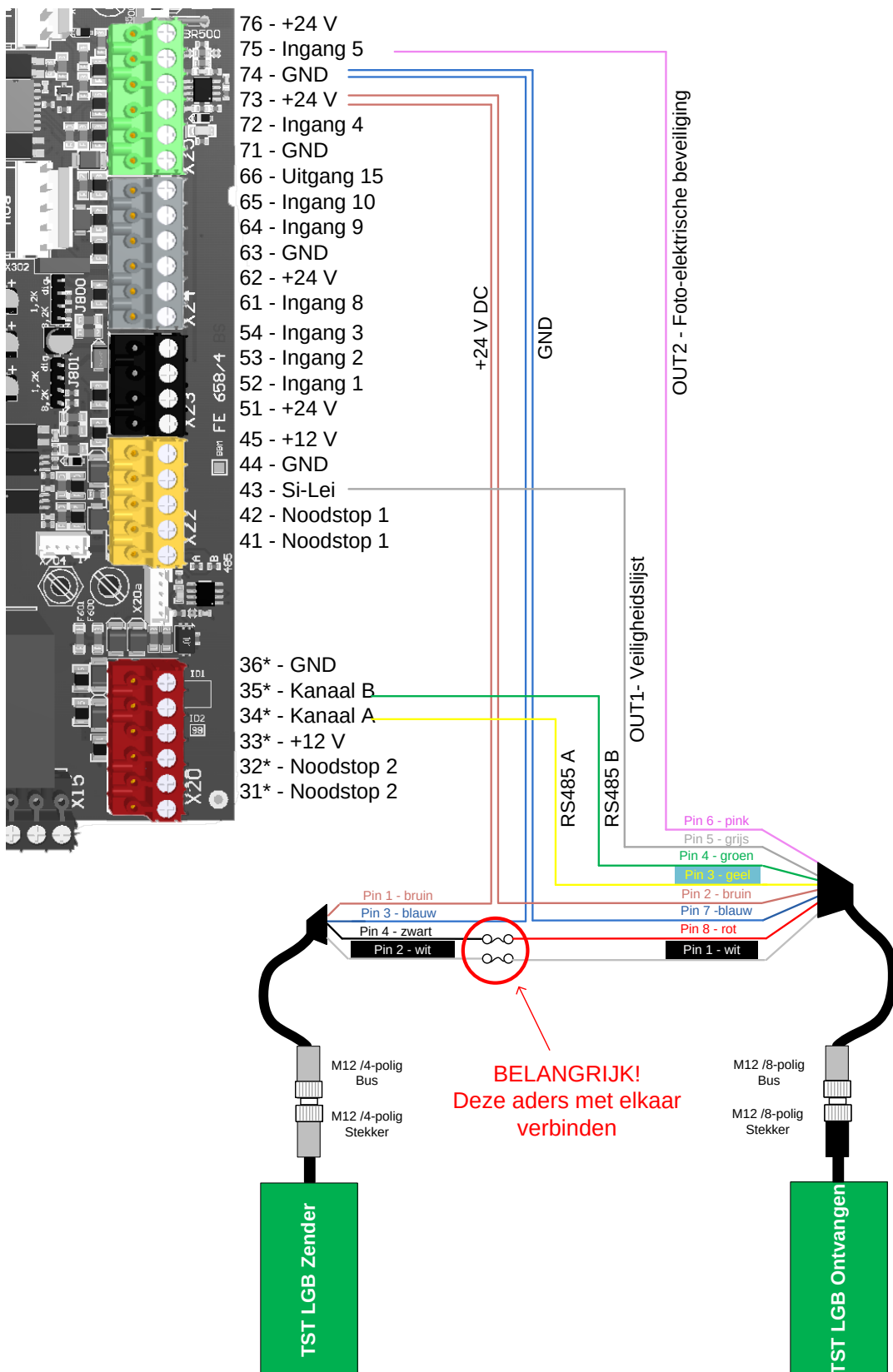
Afbeelding 17: Aansluiting TST LGB
