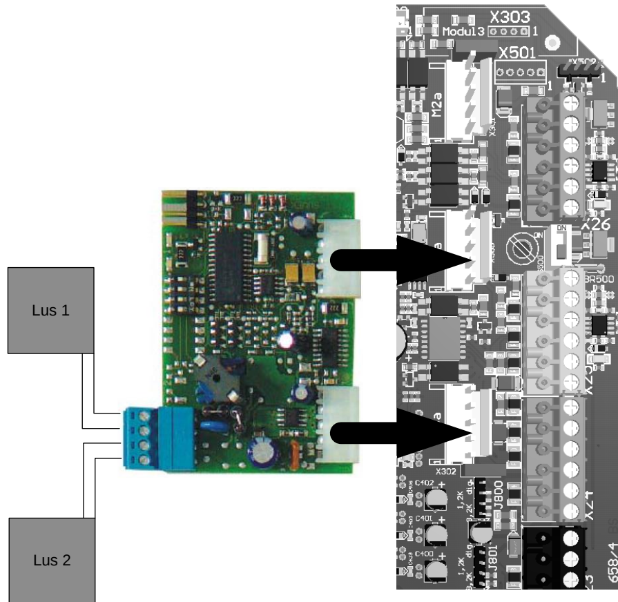
Afbeelding 28: Detectorkaart
