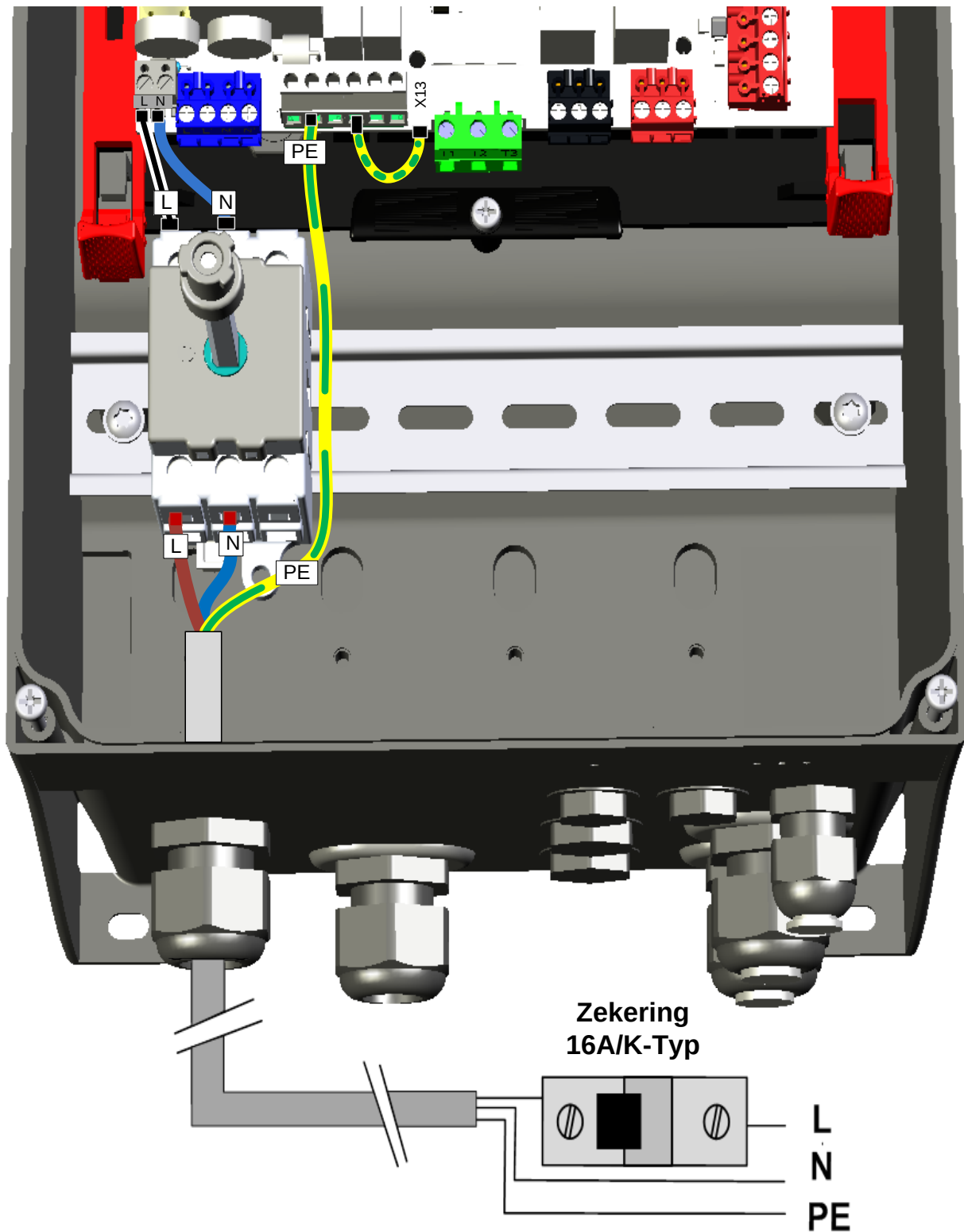
Afbeelding 9: Aansluiten van de netsnoer
