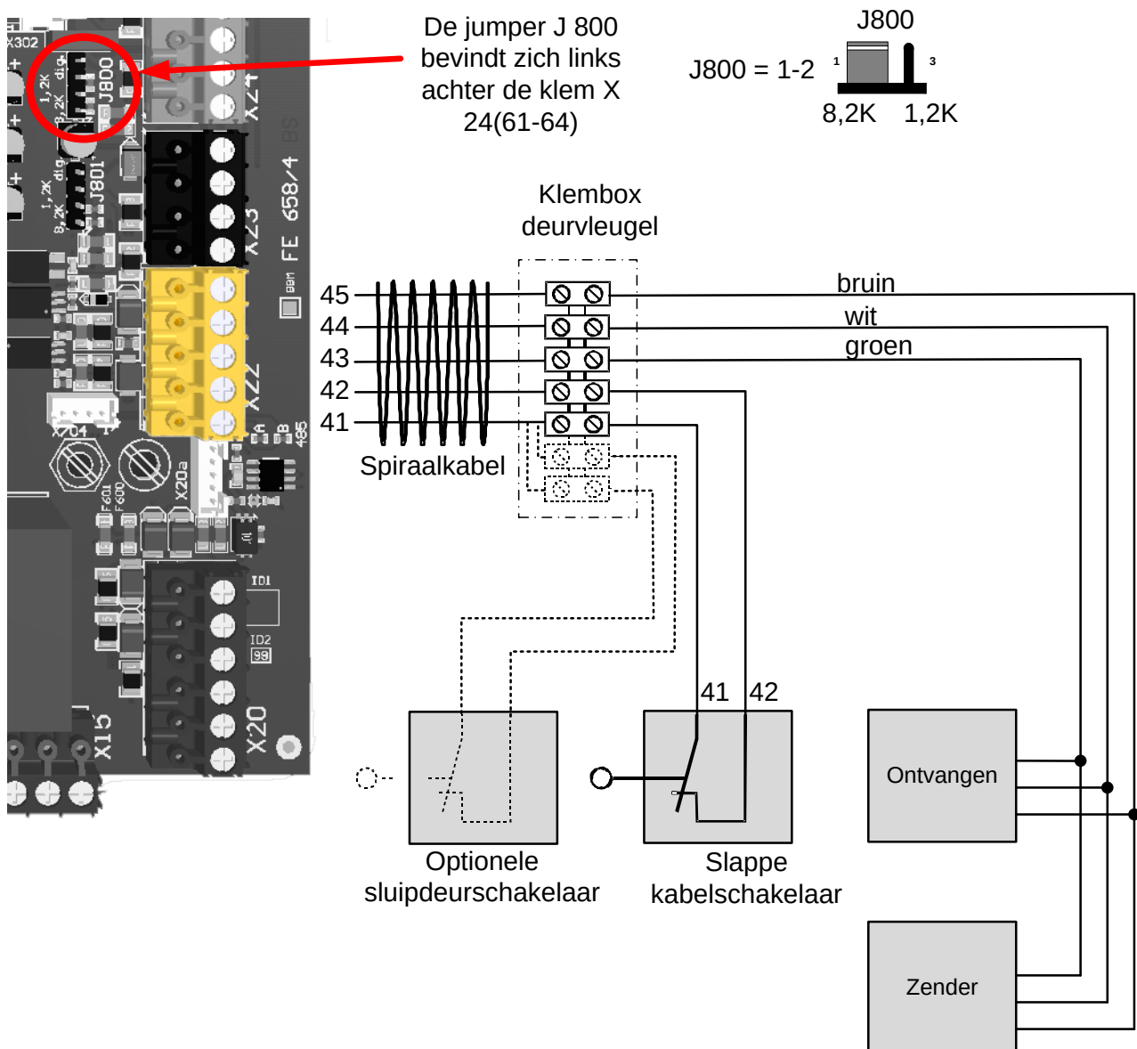
Afbeelding 11: Aansluiting optische veiligheidsstrip
