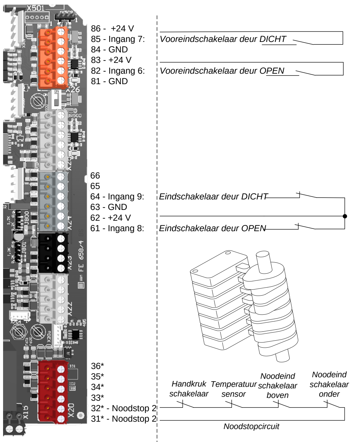
Afbeelding 21: Aansluiting noddeneindschakelaar
