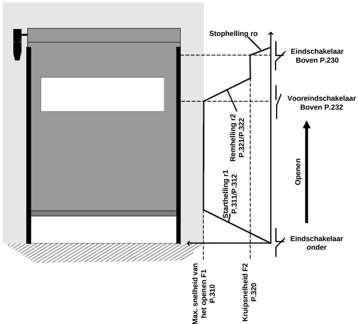
Afbeelding 39: Openen met frequentie-omzetter
