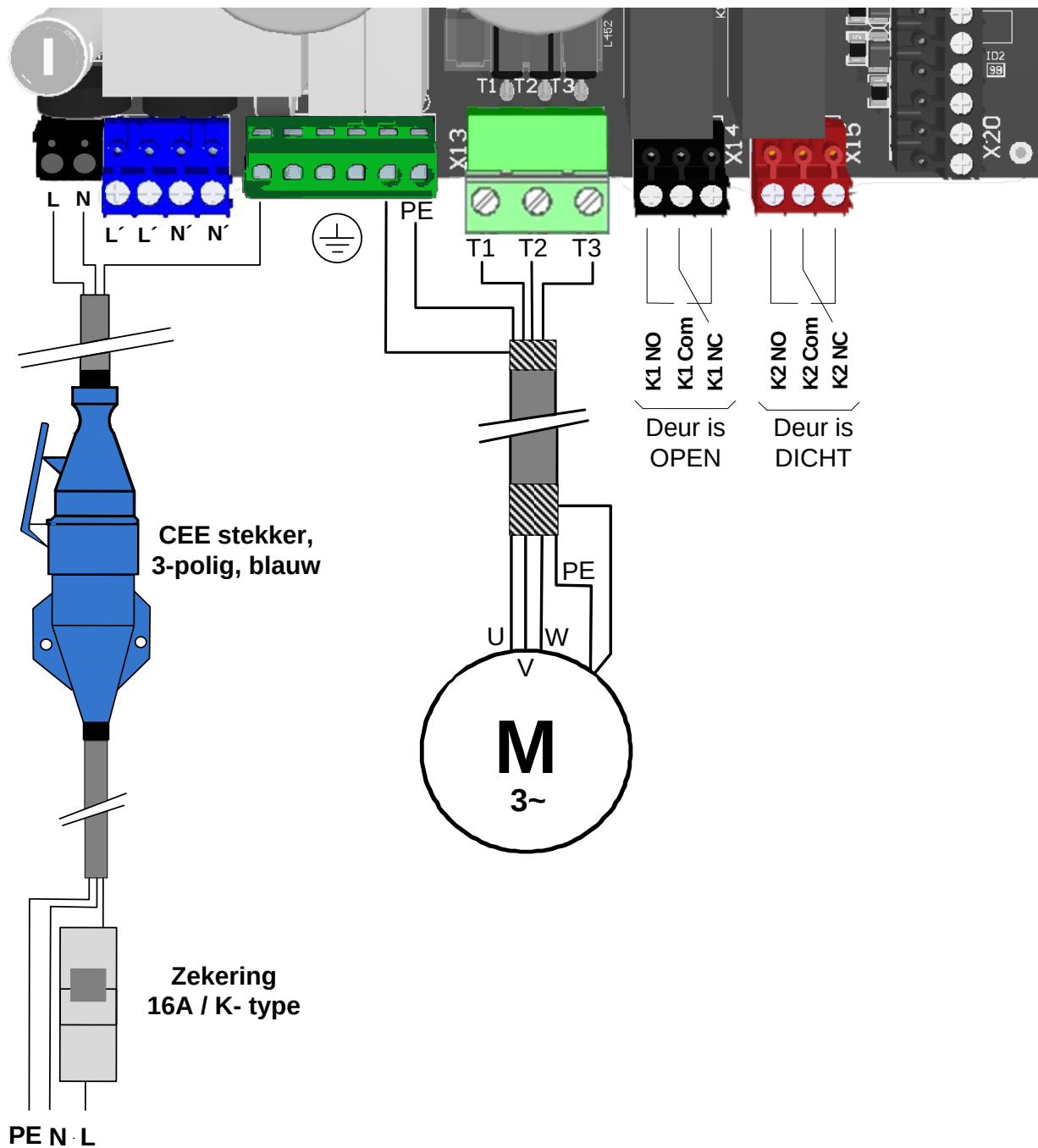
Afbeelding 25: Overzicht uitgangen
