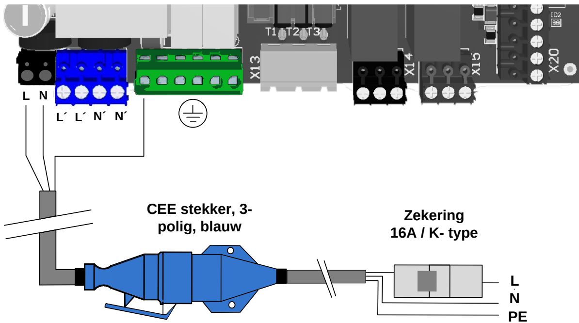
Afbeelding 8: Aansluiting netsnoer
