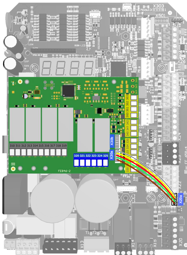
Afbeelding 34: Aansluitingsvoorbeeld met TST RFUxIO-E
