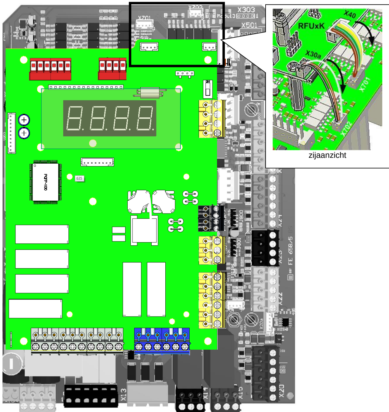
Afbeelding 31: TST RFUxK uitbreidingskaart aansluiten
