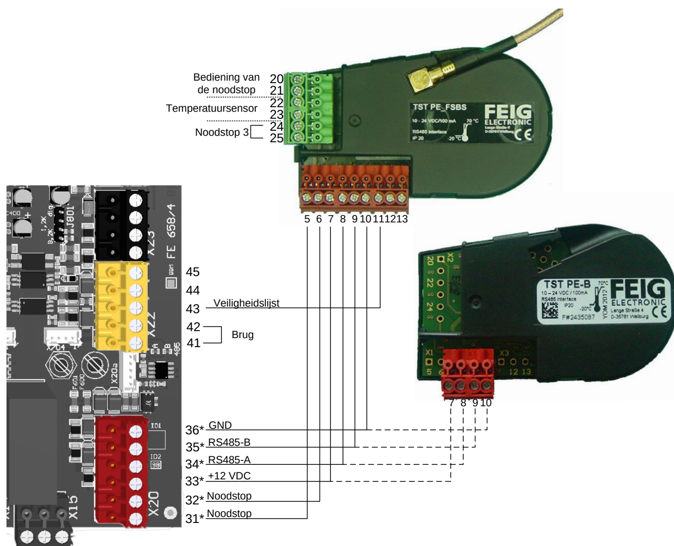
Afbeelding 18: Absolute encoder TST PE / TST PE FSB
