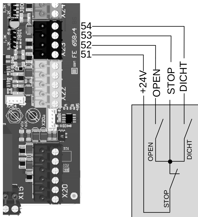
Afbeelding 23: Aansluiting van het externe commandoapparaat
