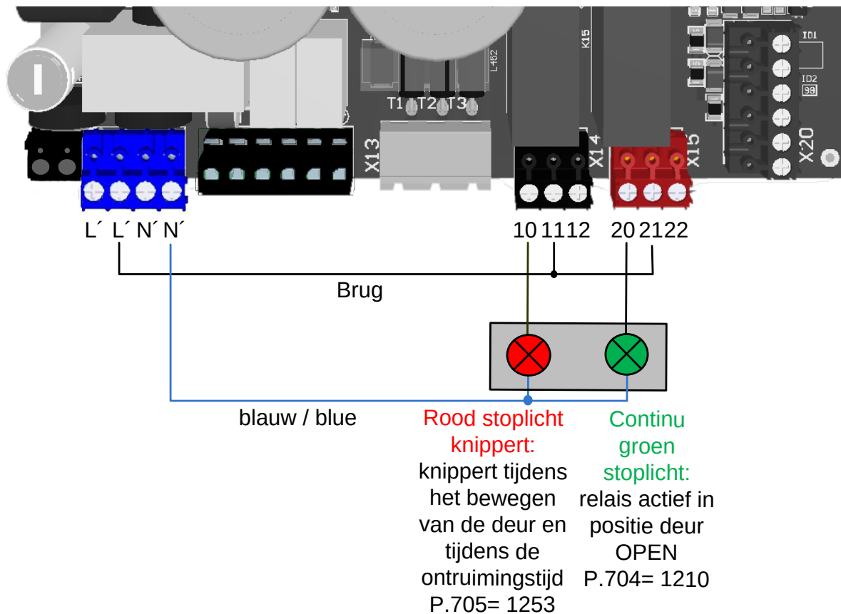
Afbeelding 24: Aansluiting van het stoplicht
