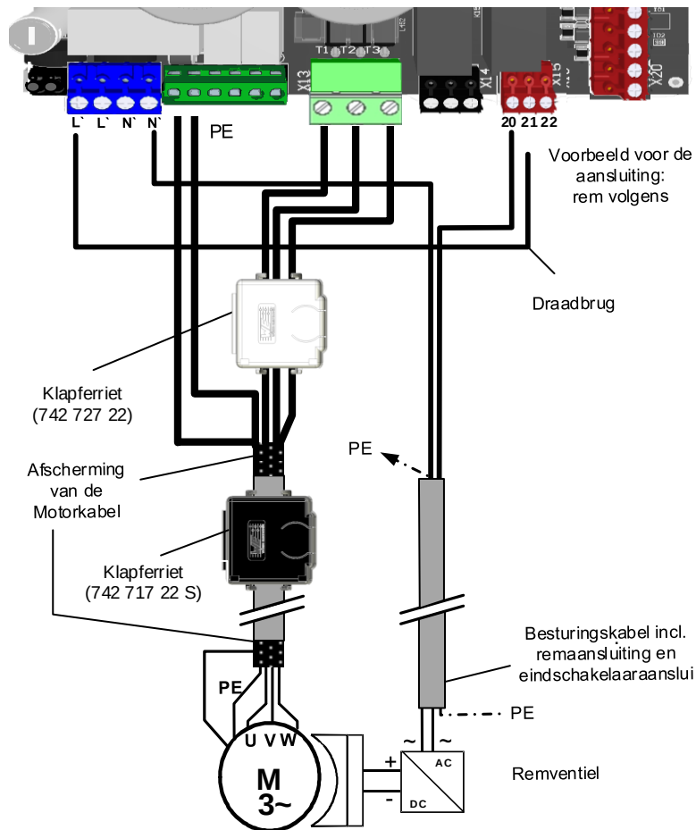
Afbeelding 10: Motoraansluiting
