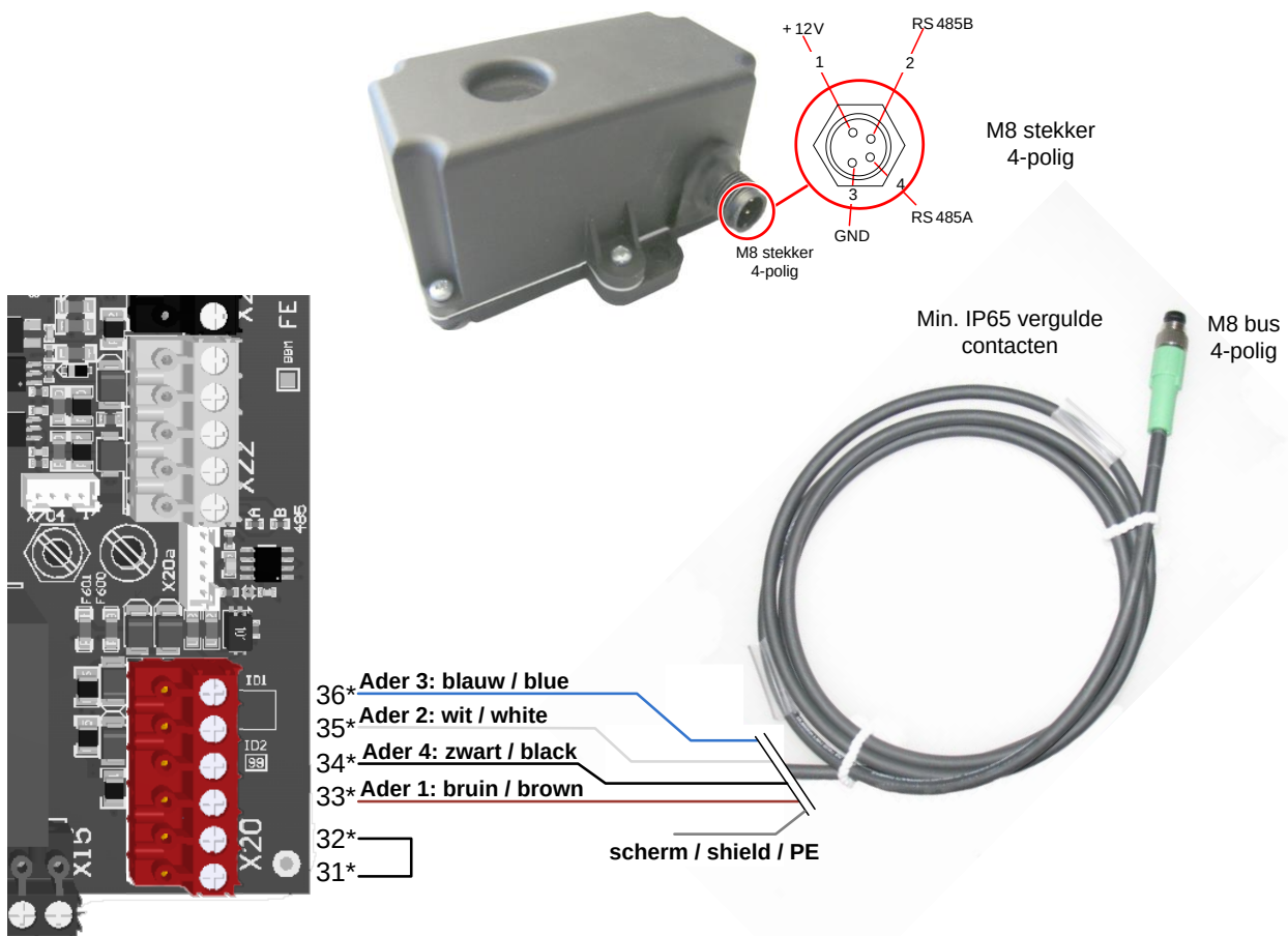
Afbeelding 19: Aansluiting van de absolute encoder TST PD
