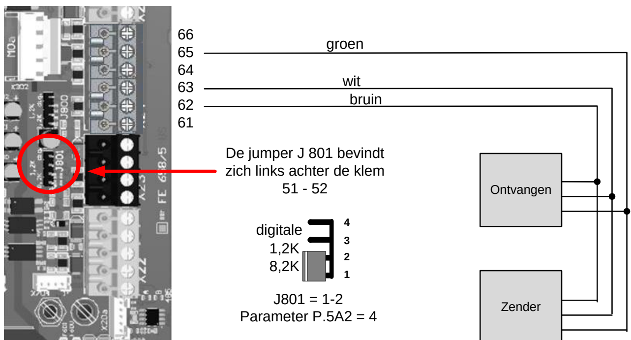
Afbeelding 13: Aansluiting optische veiligheidsstrip
