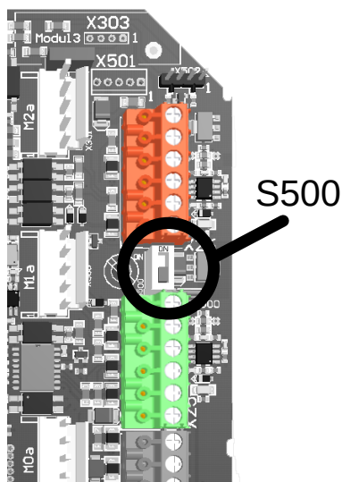
Afbeelding 36: Positie DIP- schakelaar
