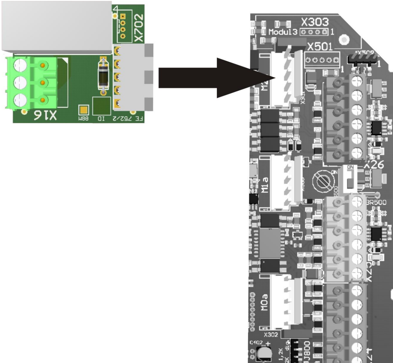
Afbeelding 33: Extra relais TST SRA
